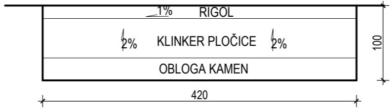
PRESJEK MJ 1:25
