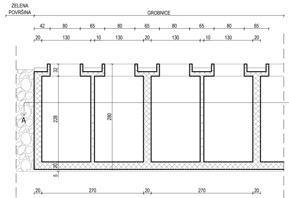
PRESJEK A-A
