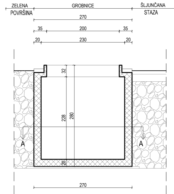
PRESJEK B-B
